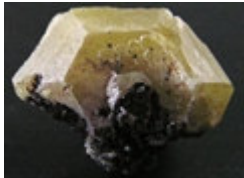
Mimetite Crystal
